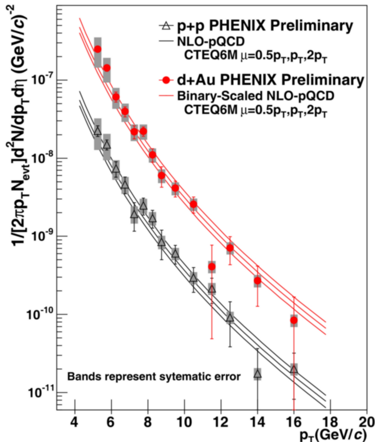
Rys. nucl-ex/0511042
