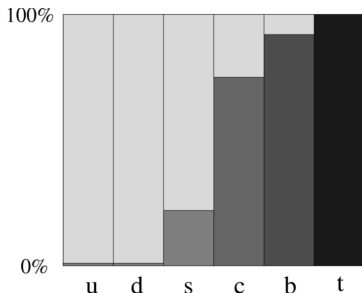
Rys. lewy: procent efektywnej masy kwarka generowanej dynamicznie (jasno szary) w porównaniu z masą z mechanizmu Higgsa w sektorze elektro-słabym Modelu Standardowego (ciemno szary), arXiv:0801.4256
